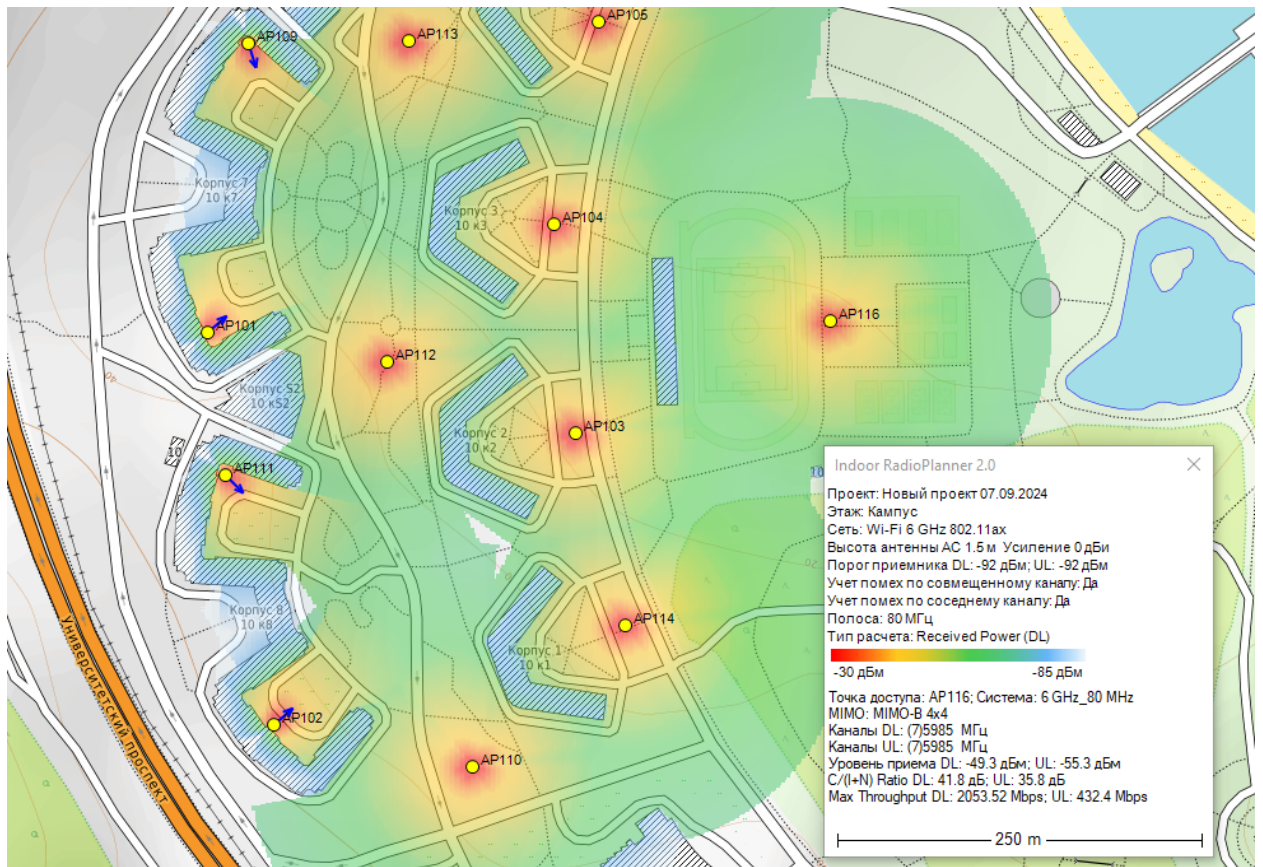
Пример расчета уровней принимаемой мощности для outdoor сети
