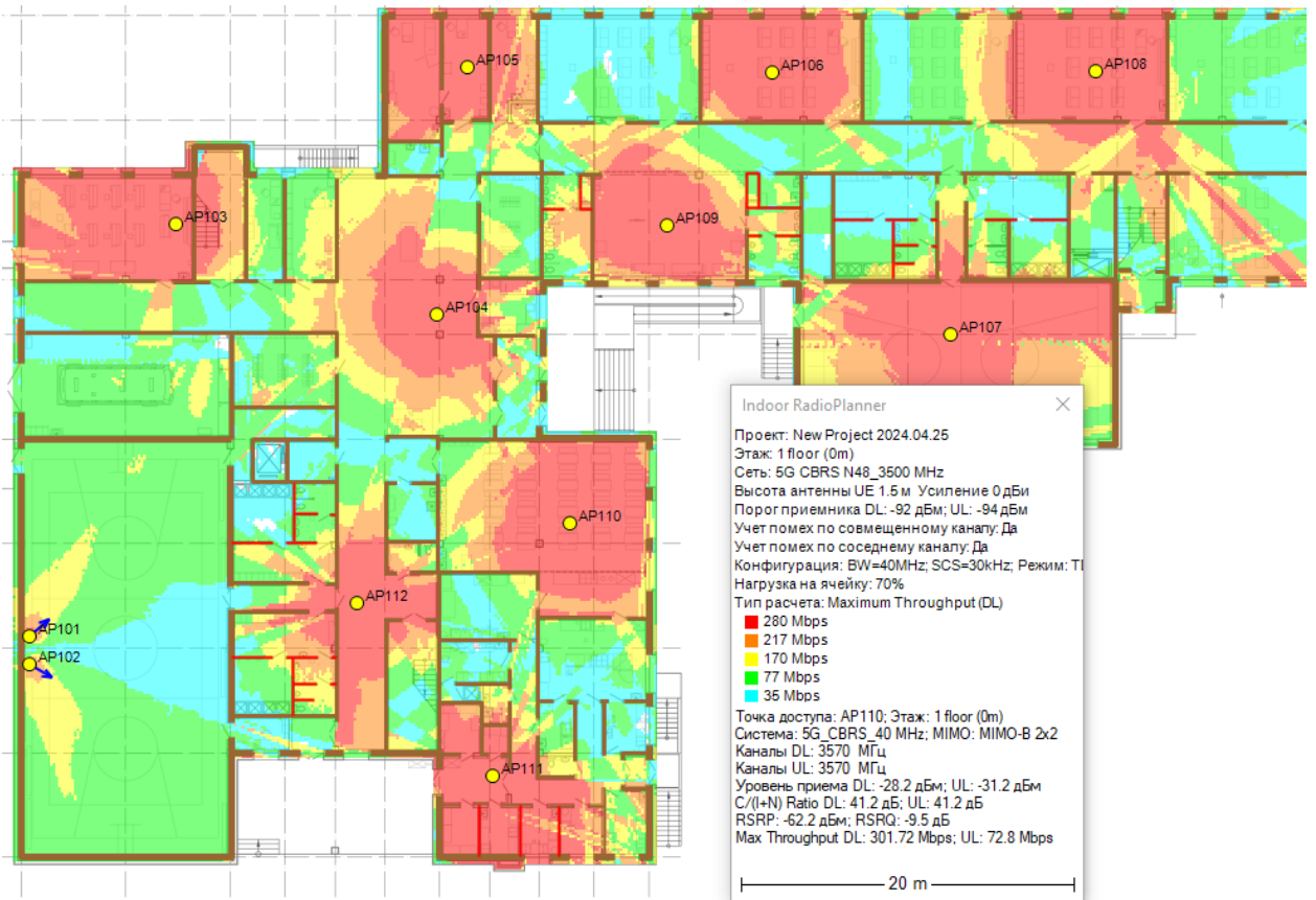
Пример расчета максимальной пропускной способности для indoor сети 5G
