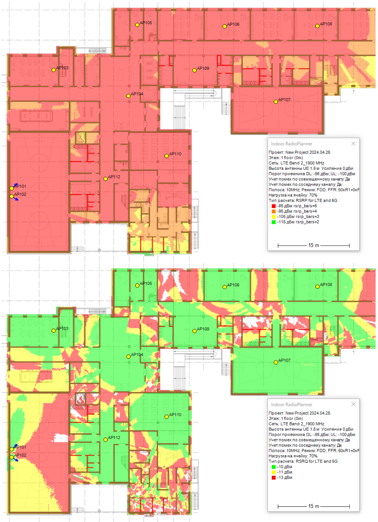
Пример расчета уровней RSRP для indoor сети LTE
