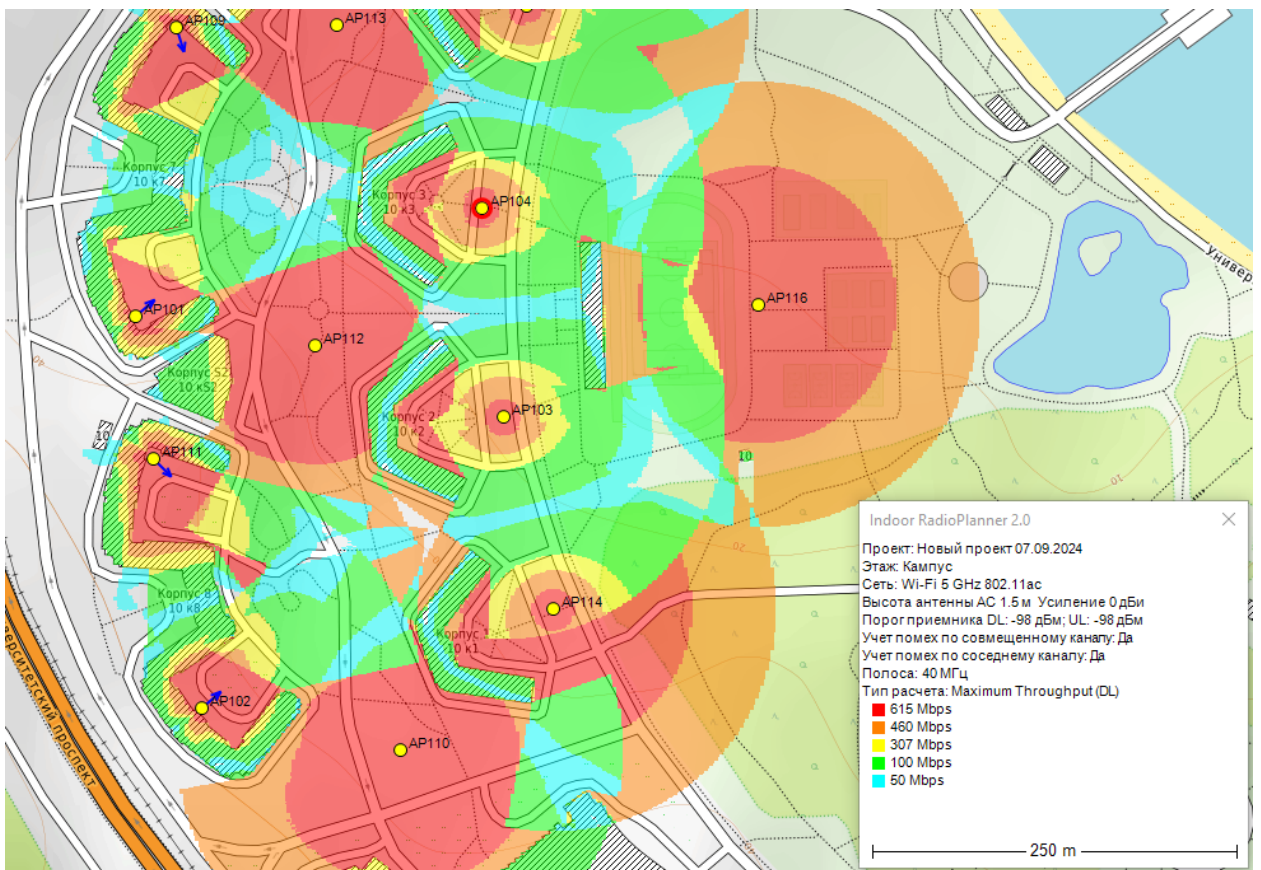
Пример расчета максимальной пропускной способности для outdoor сети Wi-Fi
