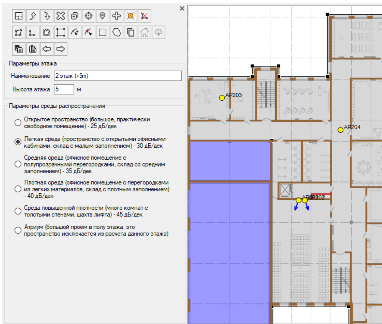
Параметры области (среды) распространения
